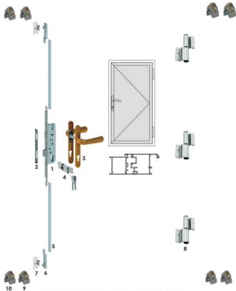
CASEMENT DOOR HARDWARE CONFIGURATION :
