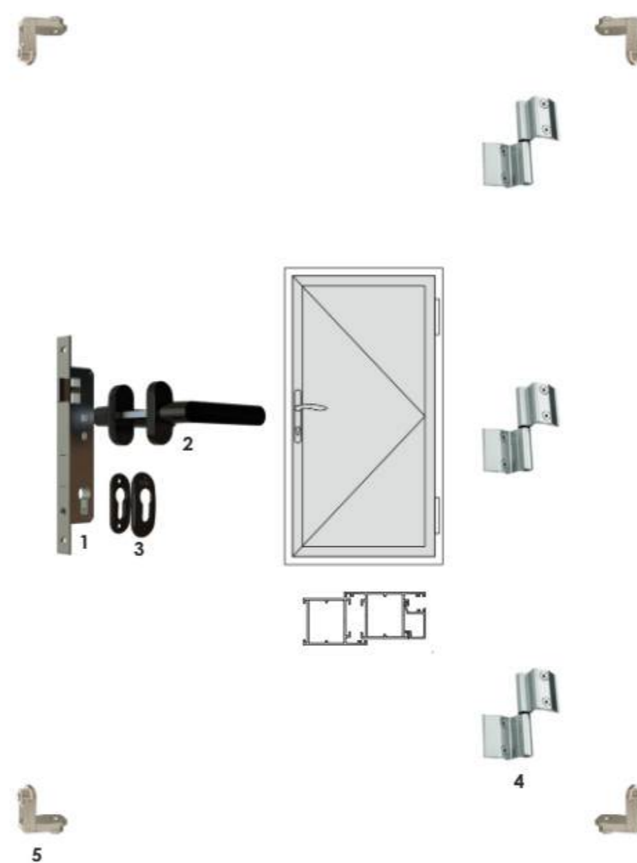
CASEMENT DOOR HARDWARE CONFIGURATION :
