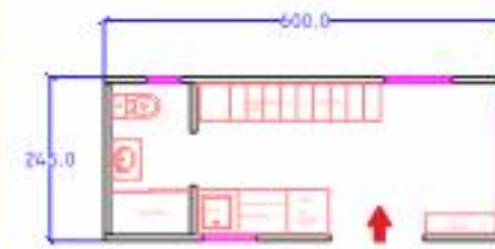
ZEMİN KAT PLANI
