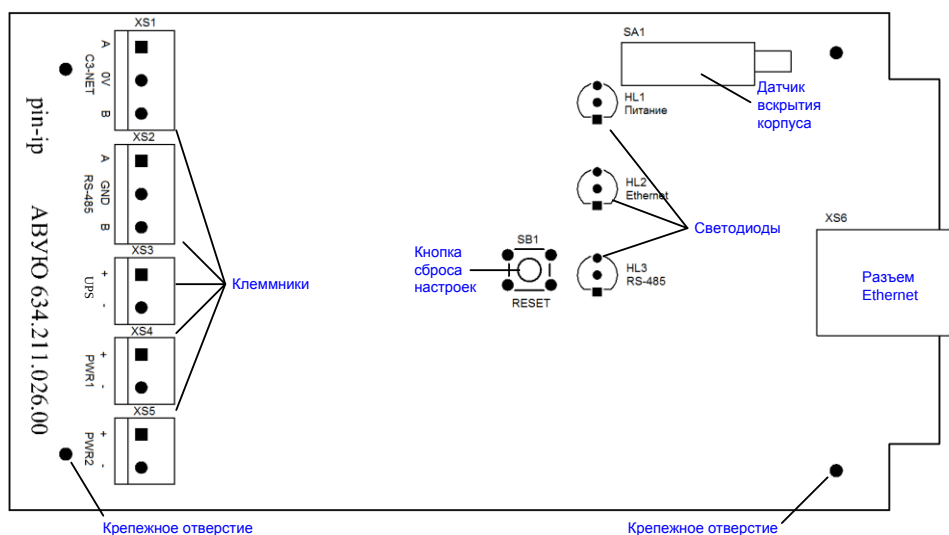
Расположение внутренних элементов ПИН-IP.
