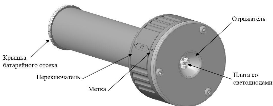
Рисунок 5. Внешний вид тестовых излучателей ИТ-12-Exd
