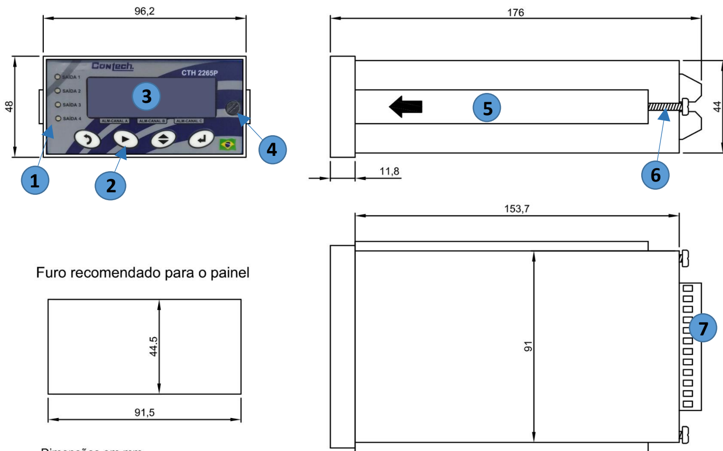
Figura 3 – Dimensões
