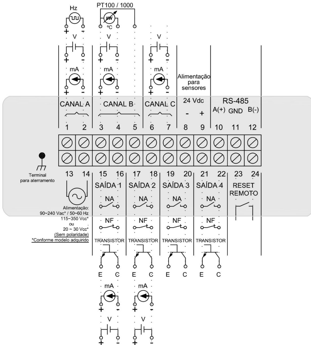
Figura 4 - Borneira traseira
