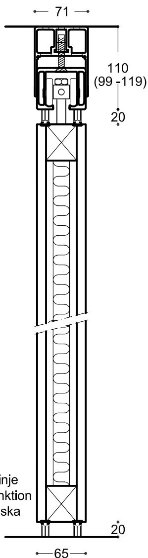
Lodrätt snitt - Rw 31-46 db - takhängd - synlig skena
