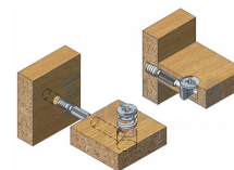
Соединение деталей эксцентриковыми стяжками
