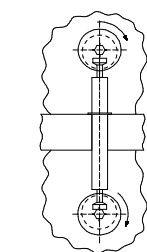
Соединение деталей двойной эксцентриковой стяжкой
