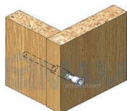
Соединение деталей евровинтами
