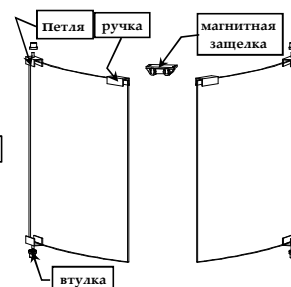
Схема установки фурнитуры на стеклянные двери
