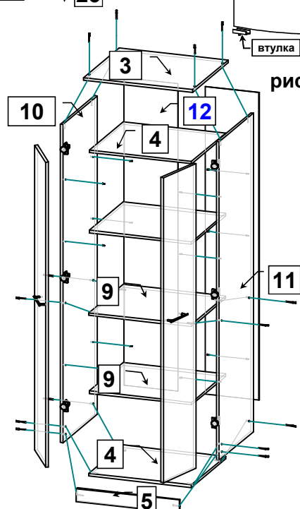
Шкаф комбинированный 06.277
