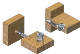
Стяжка эксцентрик
