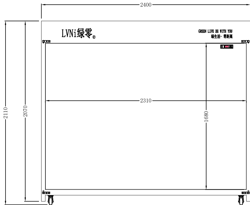
ELEVATION (前视)
