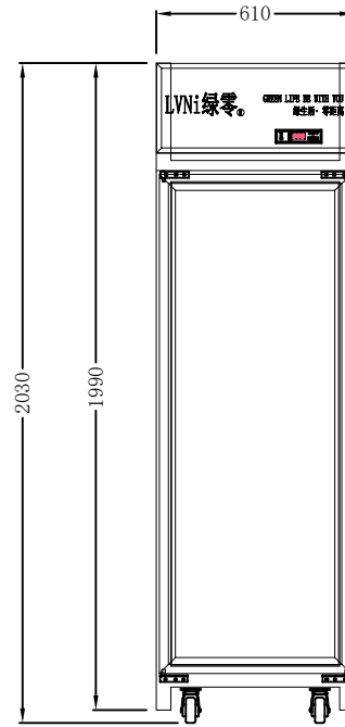
ELEVATION (前视)
