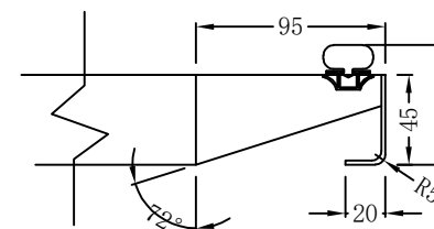
把手示意图 5:1
