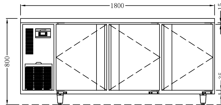
ELEVATION (前视)
