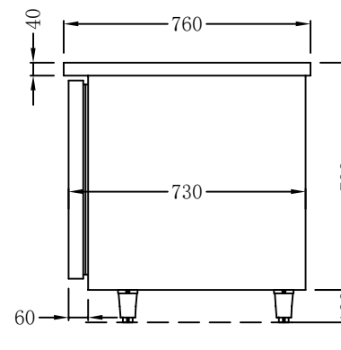
SIDE VIEW (右视)
