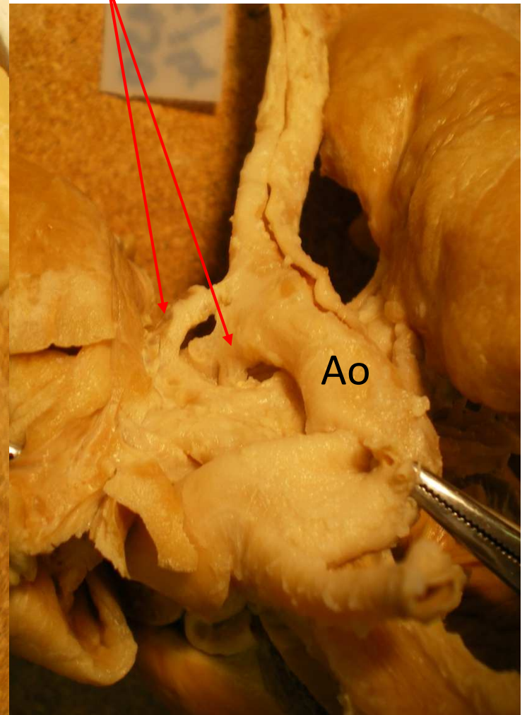
MAPCA
