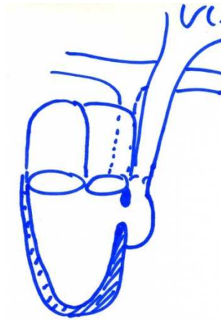
DILV {S,L,L}
