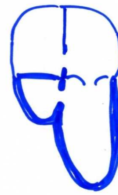
Atrésie tricuspide
