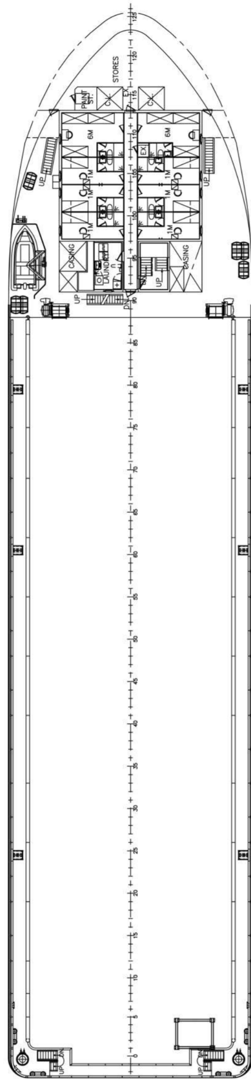
A-DECK
