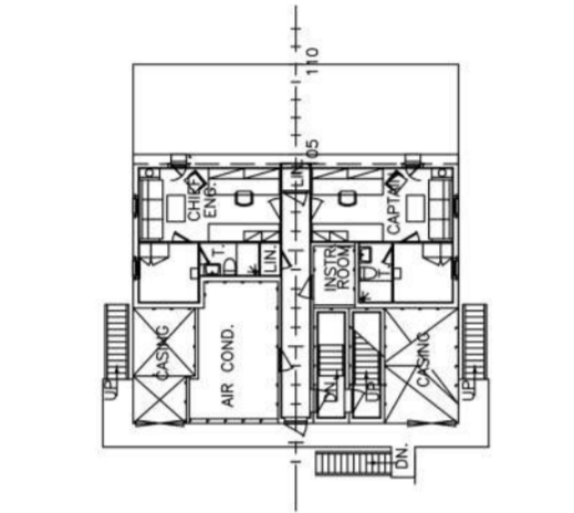
C-DECK
